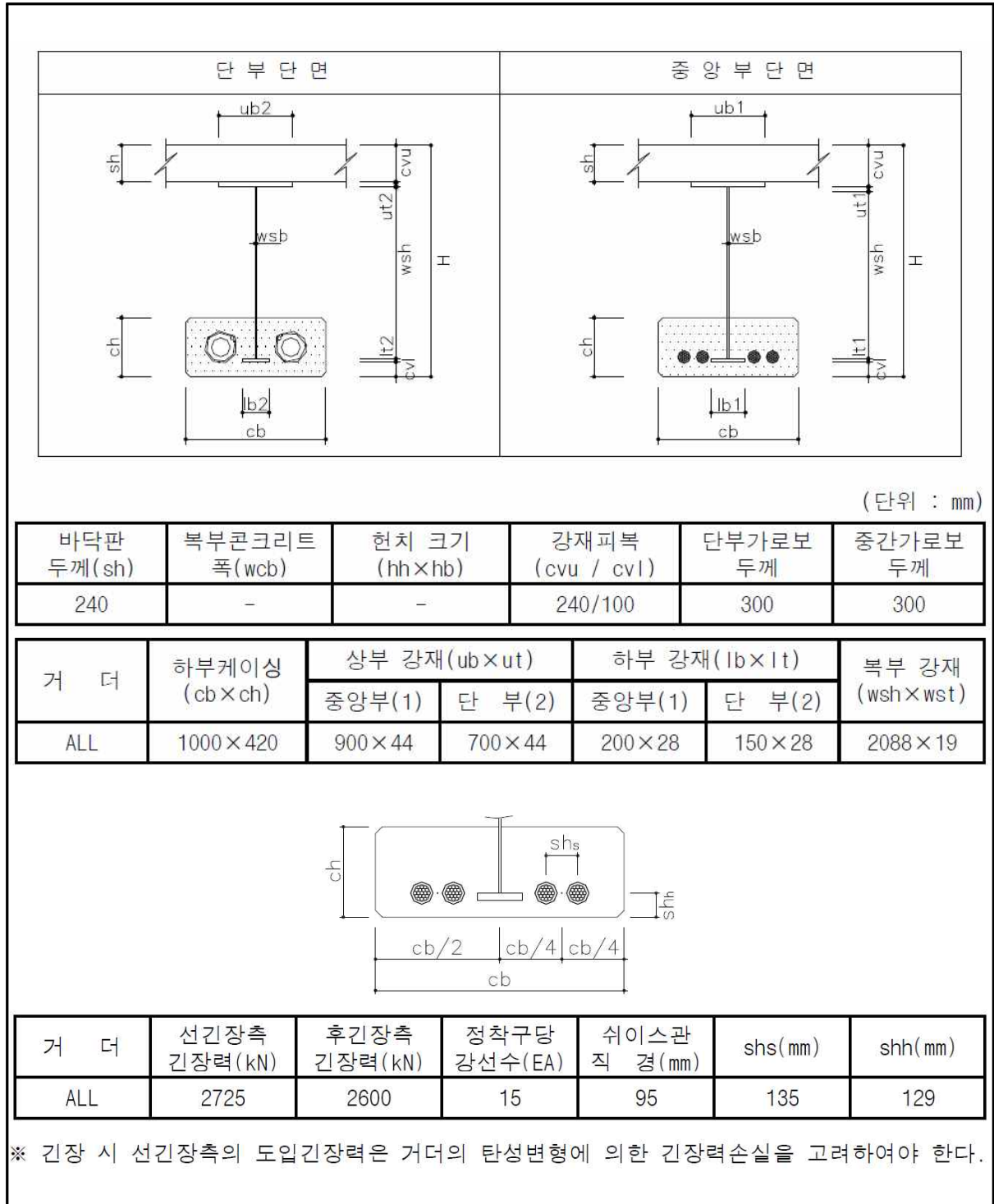
【그림 2.7.7】 해석단면
