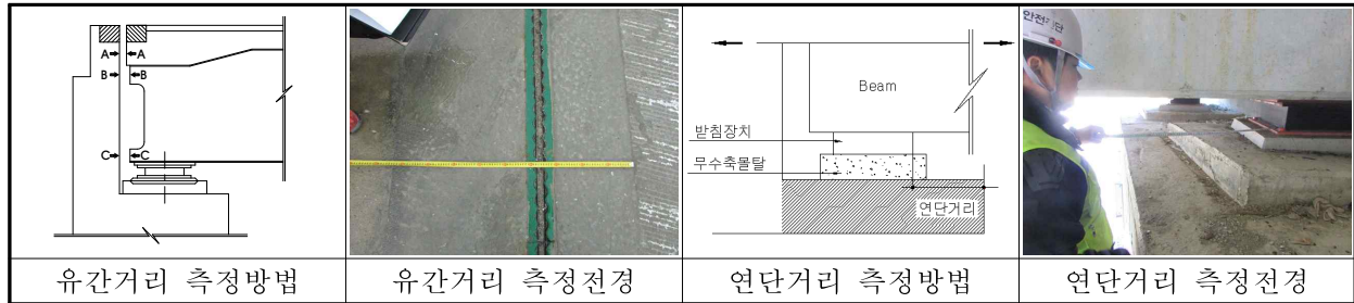
【그림 2.7.5】 부재별 기능상태 측정방법 및 전경
