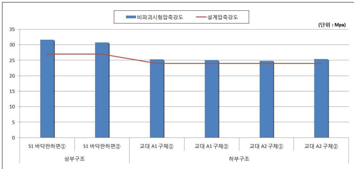
【그림 2.7.6】 콘크리트 강도시험 결과 그래프
